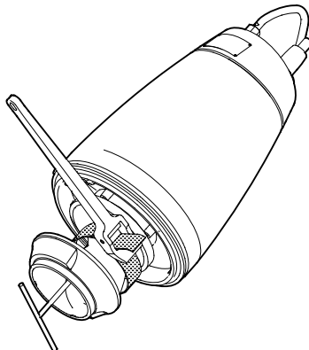
Rys. 18 Demontaż wirnika
